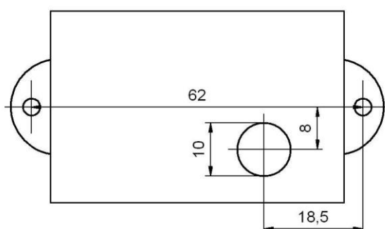
Geräteoberkante
