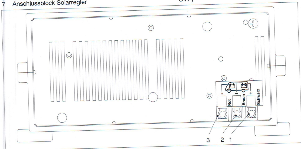
Bild 5 Aufbau Elektroblock EBL 119 (Rückseite)
