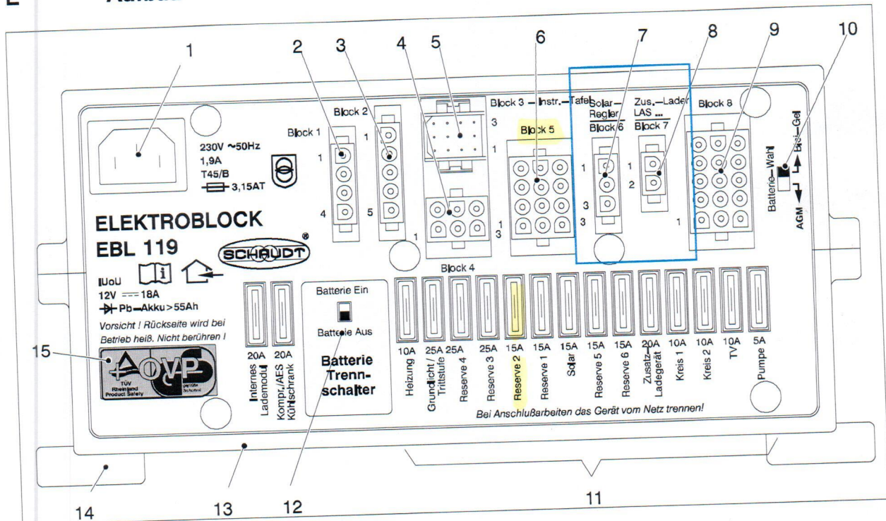
Bild 4 Aufbau Elektroblock EBL 119 (Front)
