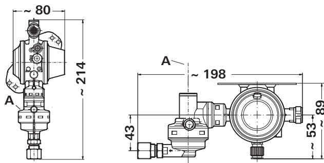
Bild 3 Maße in mm. Darstellung nicht maßstabsgerecht
