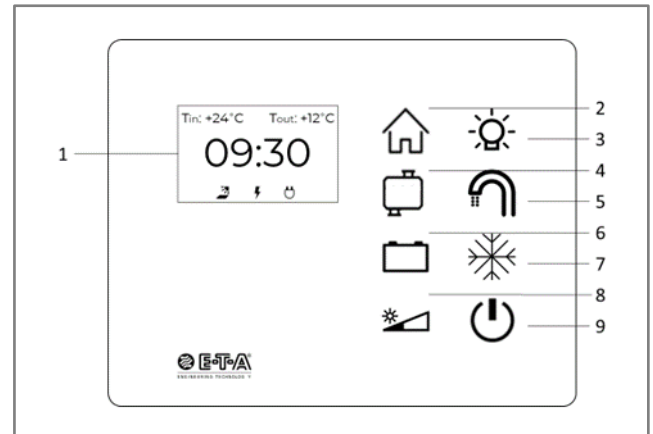
Abbildung 9: Bedienpanel D200
