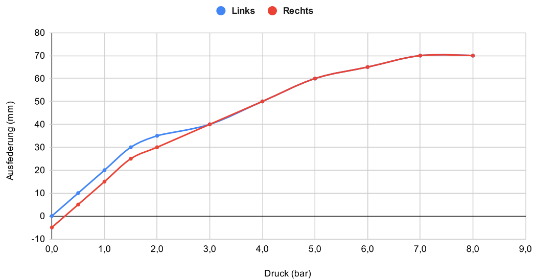
Ausfederung Zusatzluftfeder
