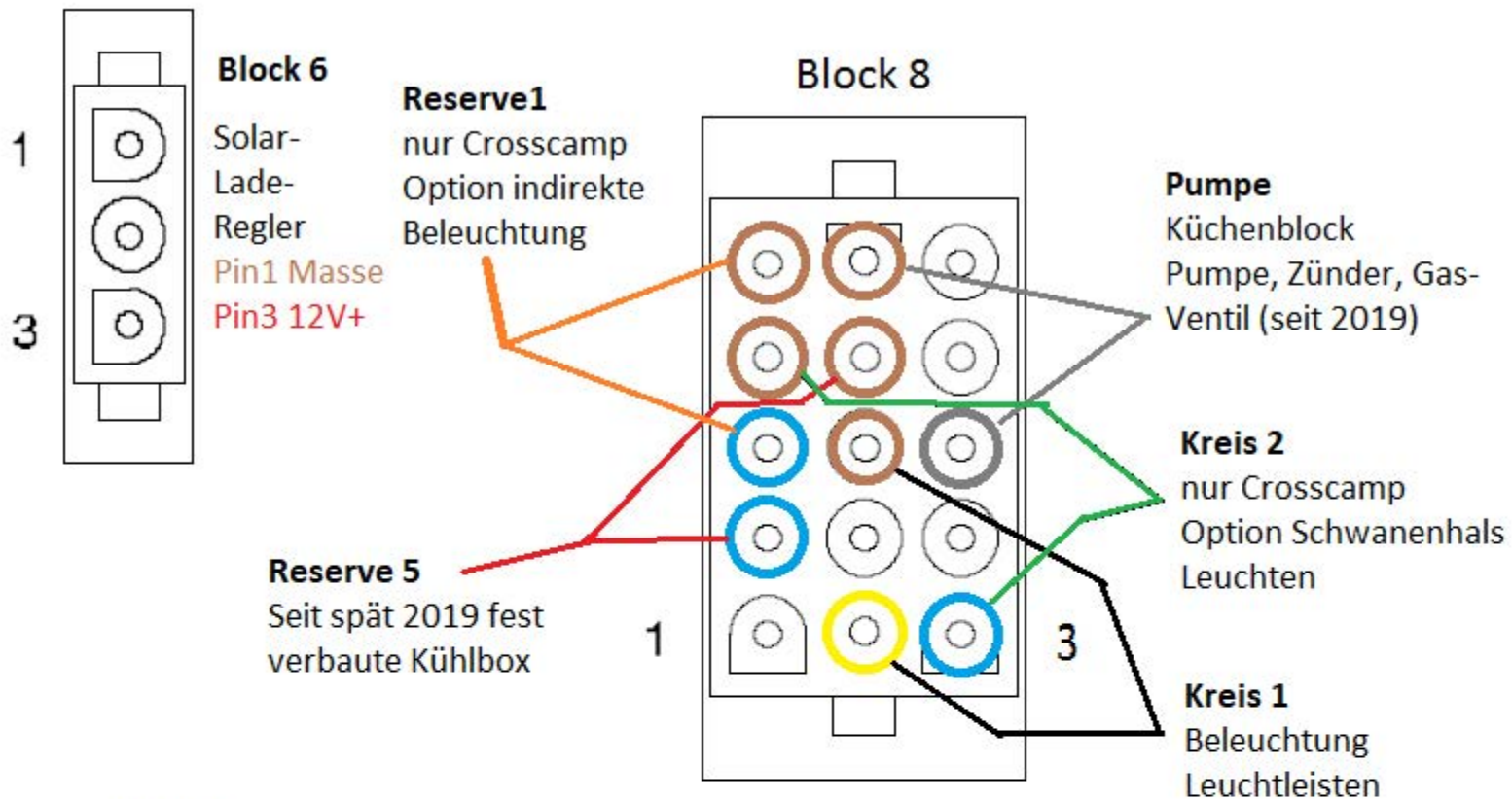
Block 4 Dauerspannung (Plug and Play 12V Steckdosen Kit)
