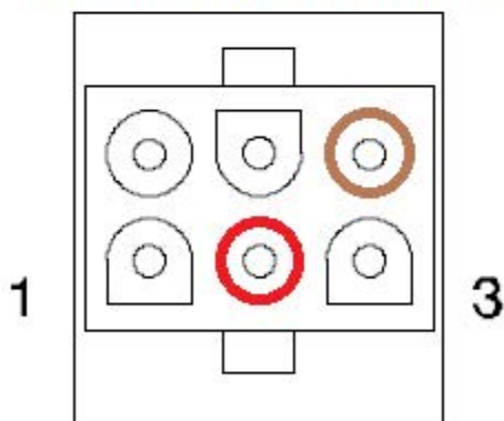
Grundlicht/Trittstufe Pin 2 und 3 12V+ Pin 6 Masse
