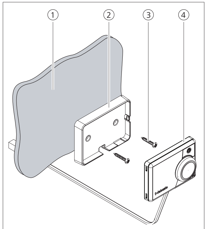
Fig. 03: Bedienelement mit Halter einbauen
