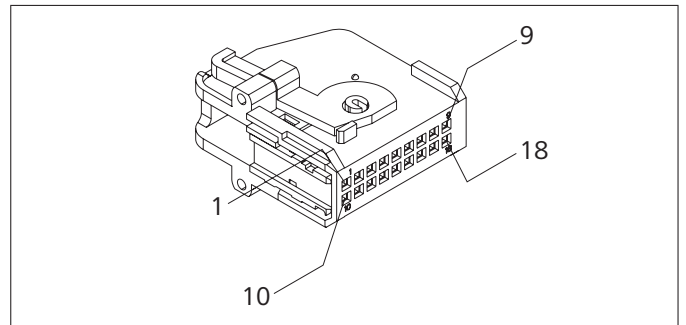
Fig. 19: Anschlüsse UniBox
