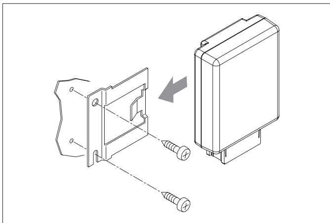
Fig. 05: Optional: UniBox mit Halter einbauen
