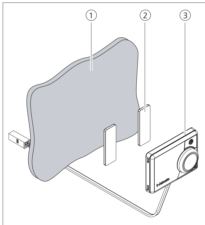
Fig. 02: Bedienelement mit Klebepads einbauen
